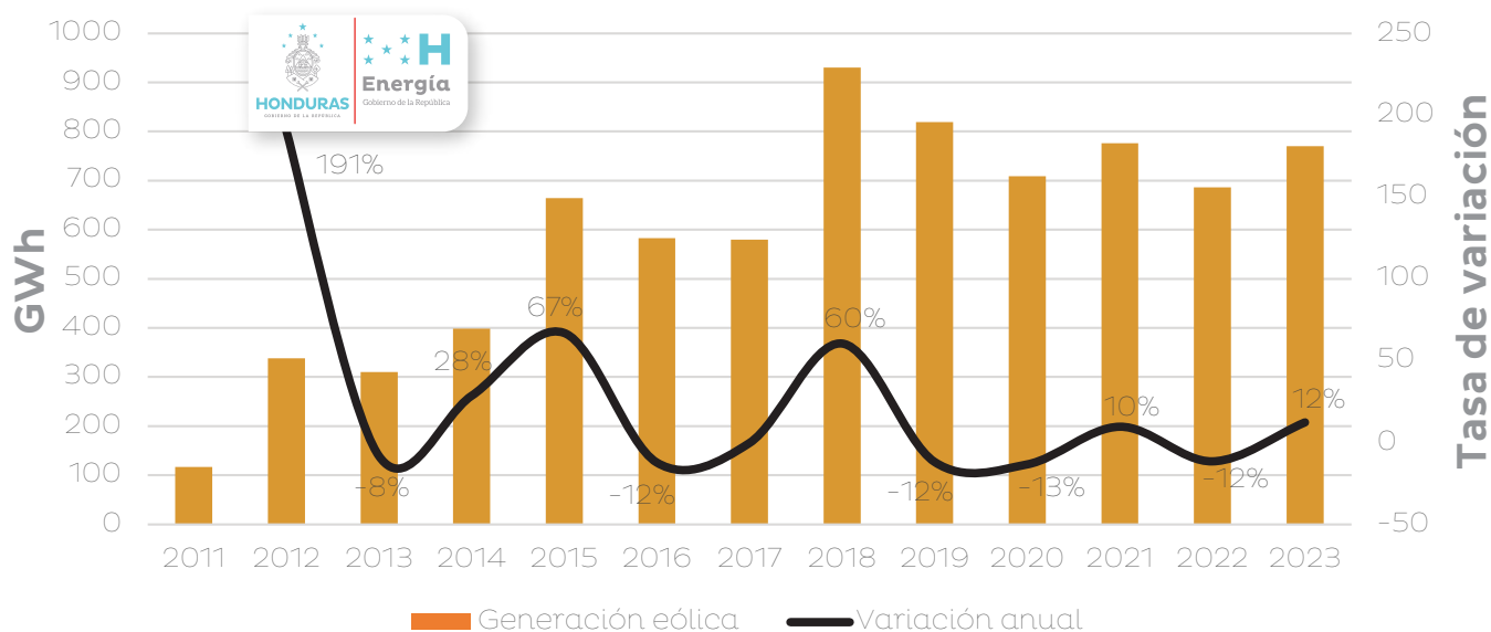
Figura 7: Generación eólica bruta (GWh)
