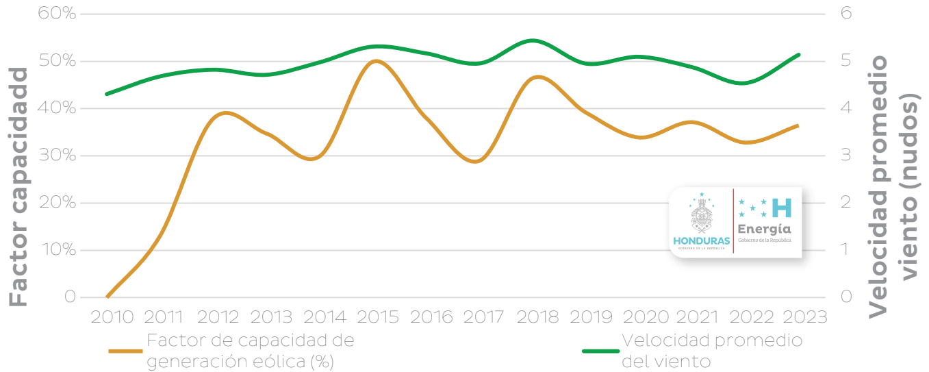
Figura 8: Factor de capacidad de generación eólica y velocidad promedio de viento
