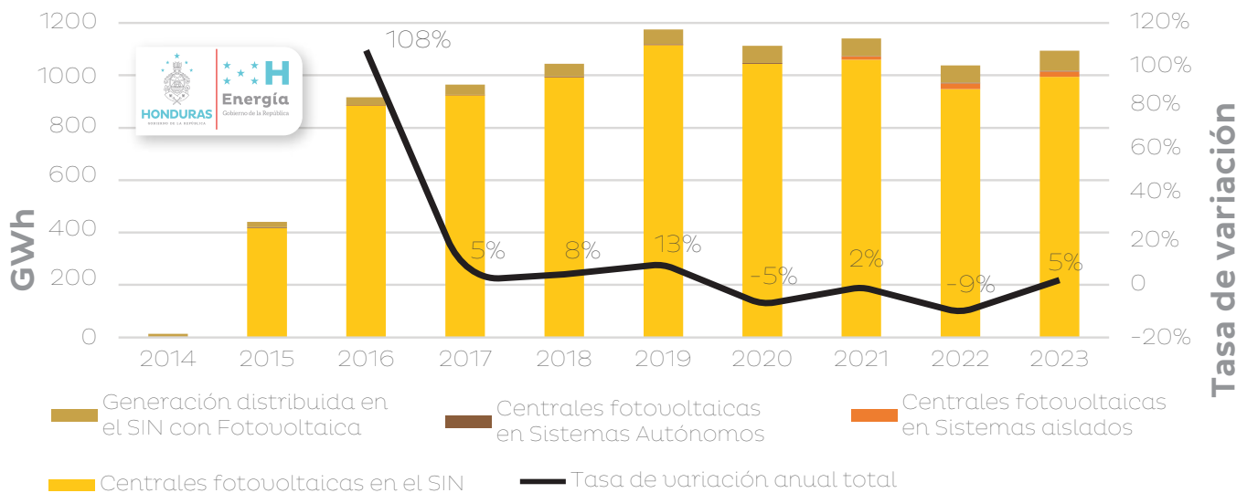
Figura 12: Generación fotovoltaica bruta (GWh)
