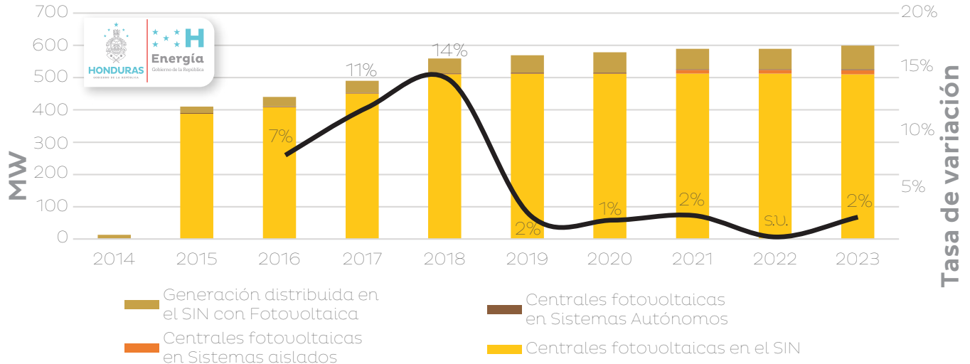
Figura 11: Capacidad fotovoltaica instalada (MW)
