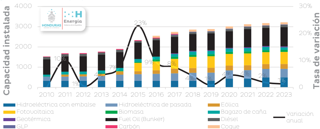
Figura 25: Capacidad instalada por tipo de recurso
