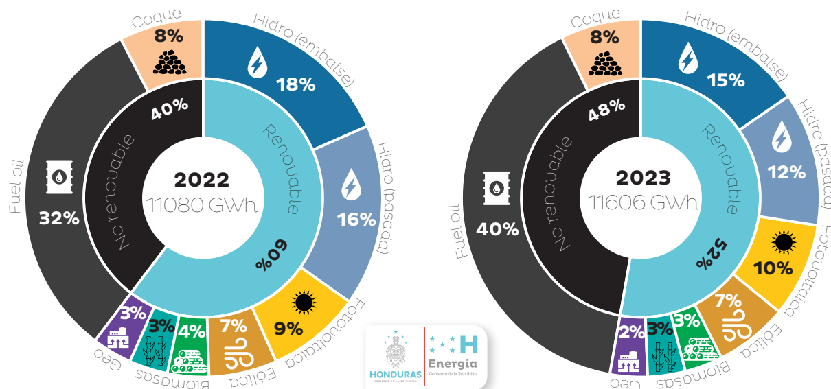
Figura 29: Comparación generación eléctrica en el SIN 2022-2023
