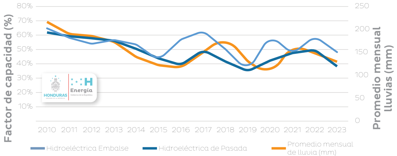
Figura 5: Factor de capacidad de la generación hidroeléctrica y promedio mensual de lluvias
