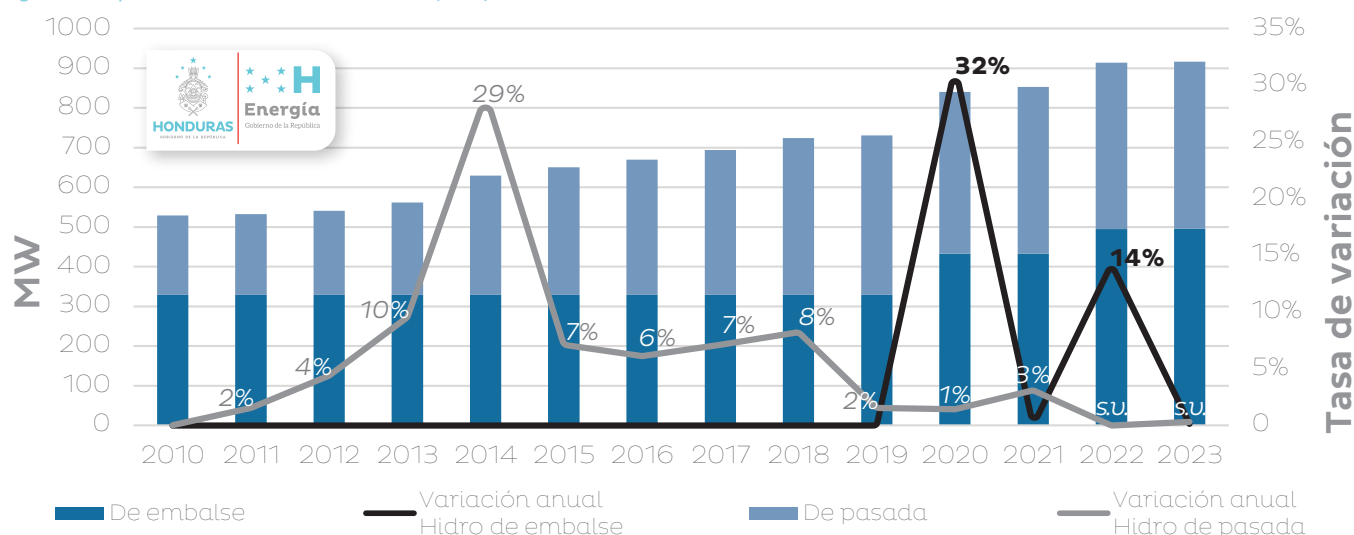
Figura 3: Capacidad hidroeléctrica instalada (MW)
