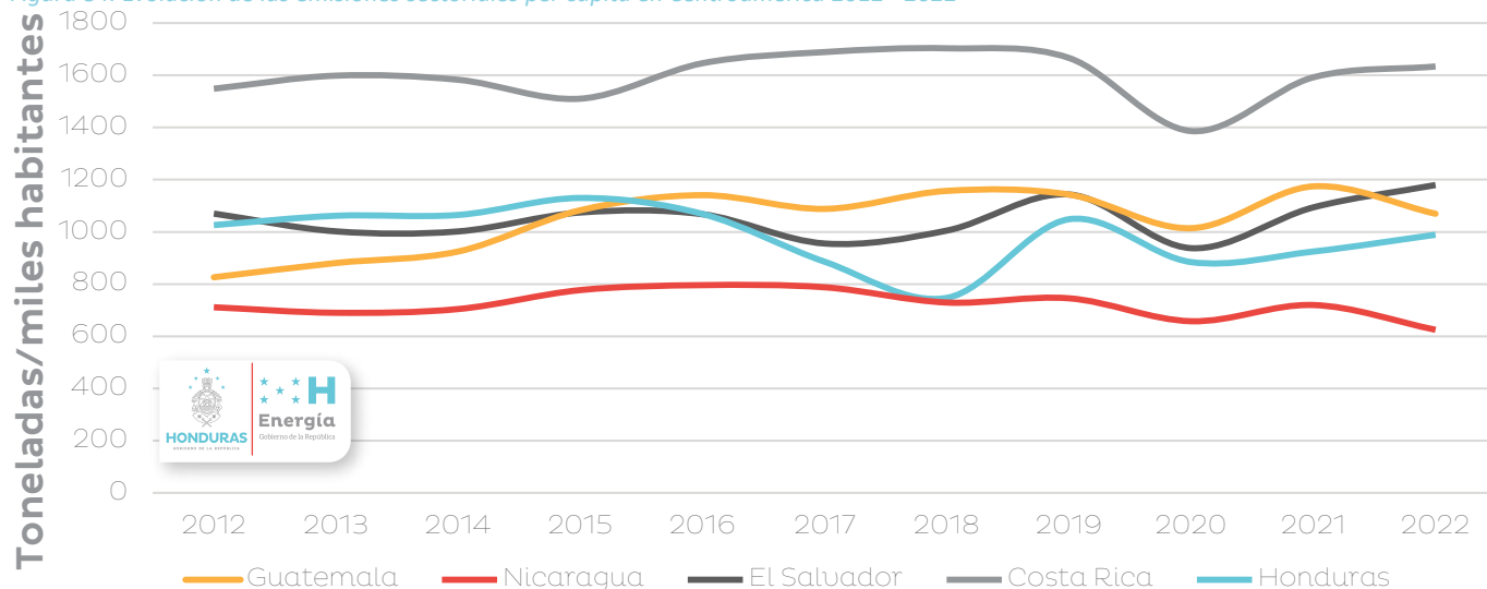
Figura 84. Evolución de las emisiones sectoriales per cápita en Centroamérica 2012 - 2022
