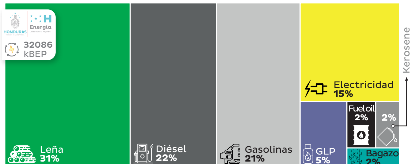
Figura 64. Demanda según energético durante el 2023
