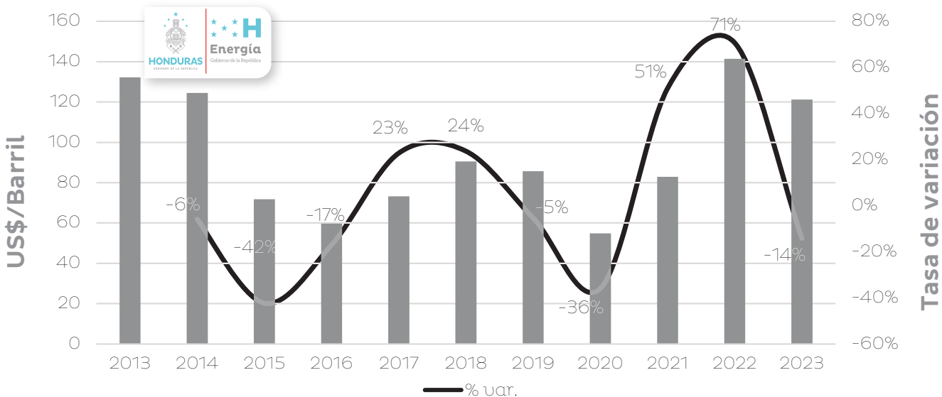
Figura 46. Precio promedio de importación del Kerosene
