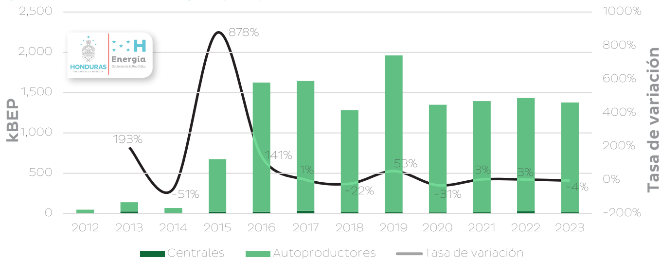
Figura 23. Consumo de combustibles vegetales para el periodo 2012 - 2023
