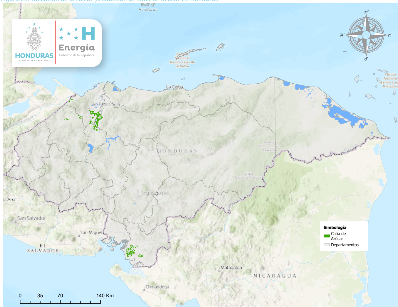
Figura 20. Ubicación de áreas de producción de caña de azúcar en Honduras
