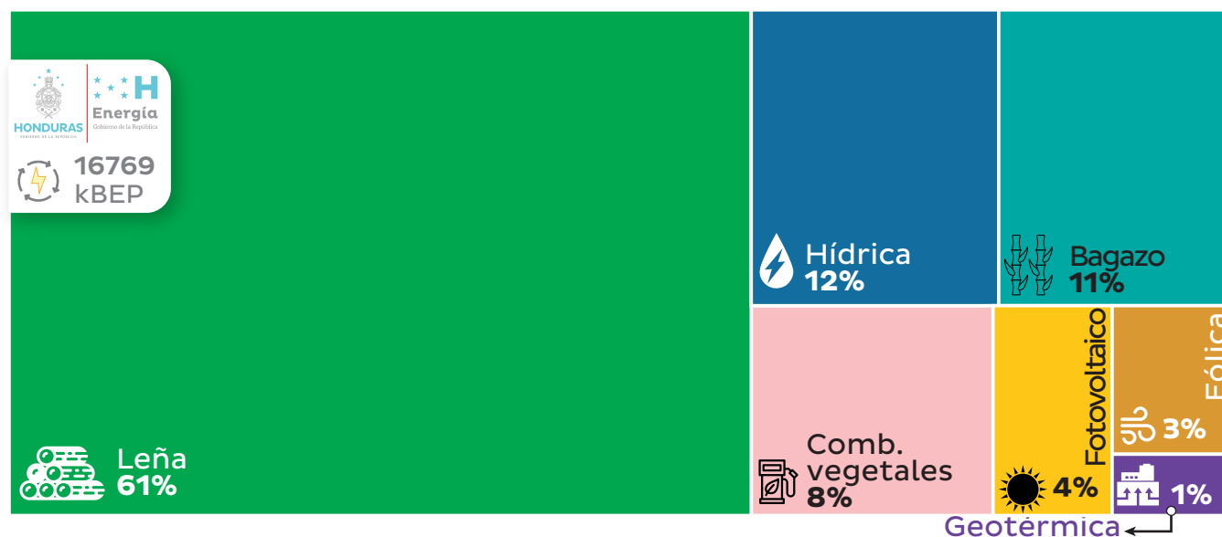
Figura 61. Oferta de energías primarias durante el 2023
