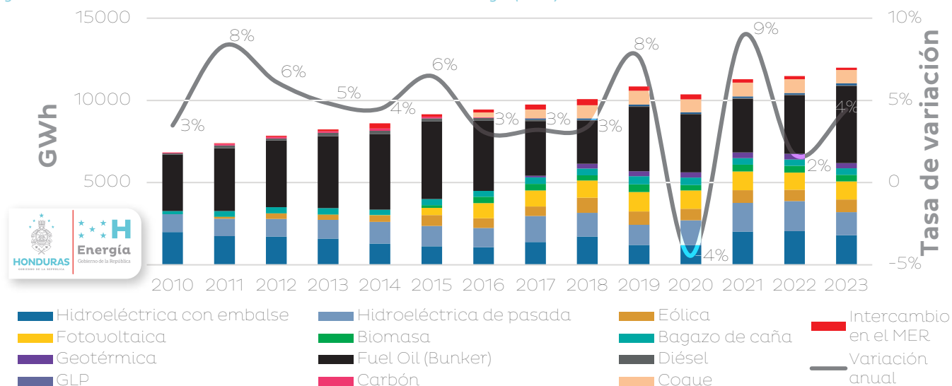
Figura 26: Generación de electricidad en Honduras e intercambio de energía (GWh)
