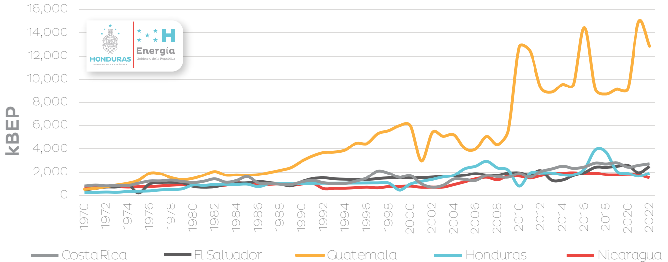
Figura 19. Oferta de bagazo en Centroamérica 1970 – 2022
