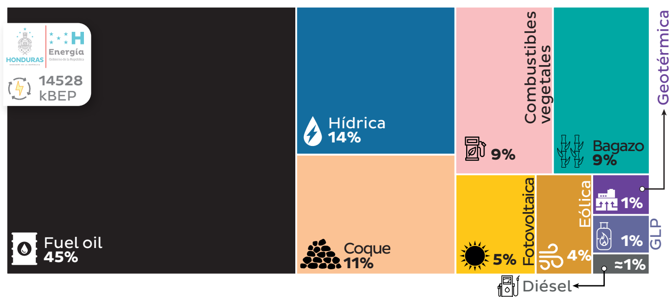
Figura 63. Insumos energéticos para los centros de transformación
