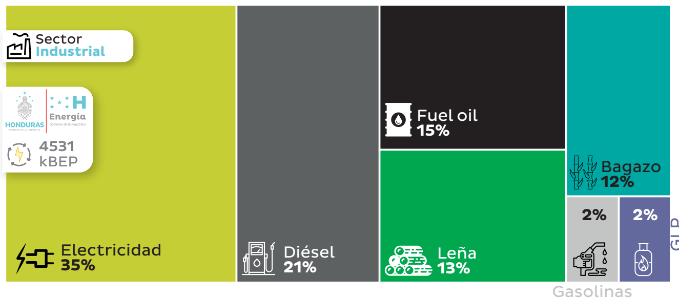
Figura 67. Demanda energética en el sector industrial
