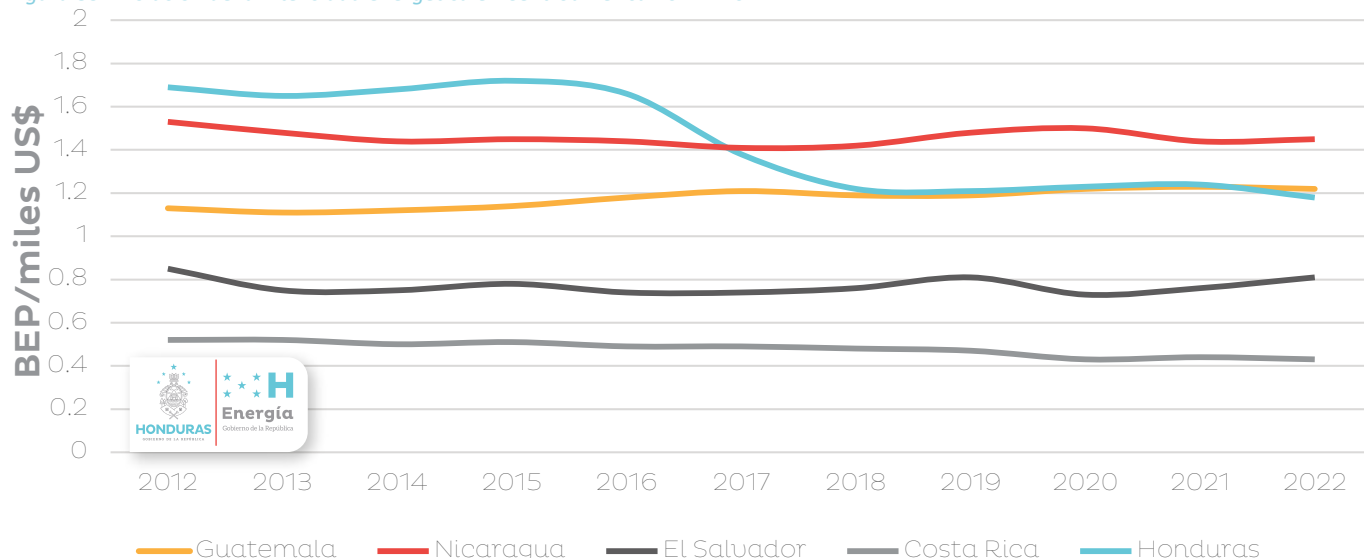
Figura 83. Evolución de la intensidad energética en Centroamérica 2012 - 2022
