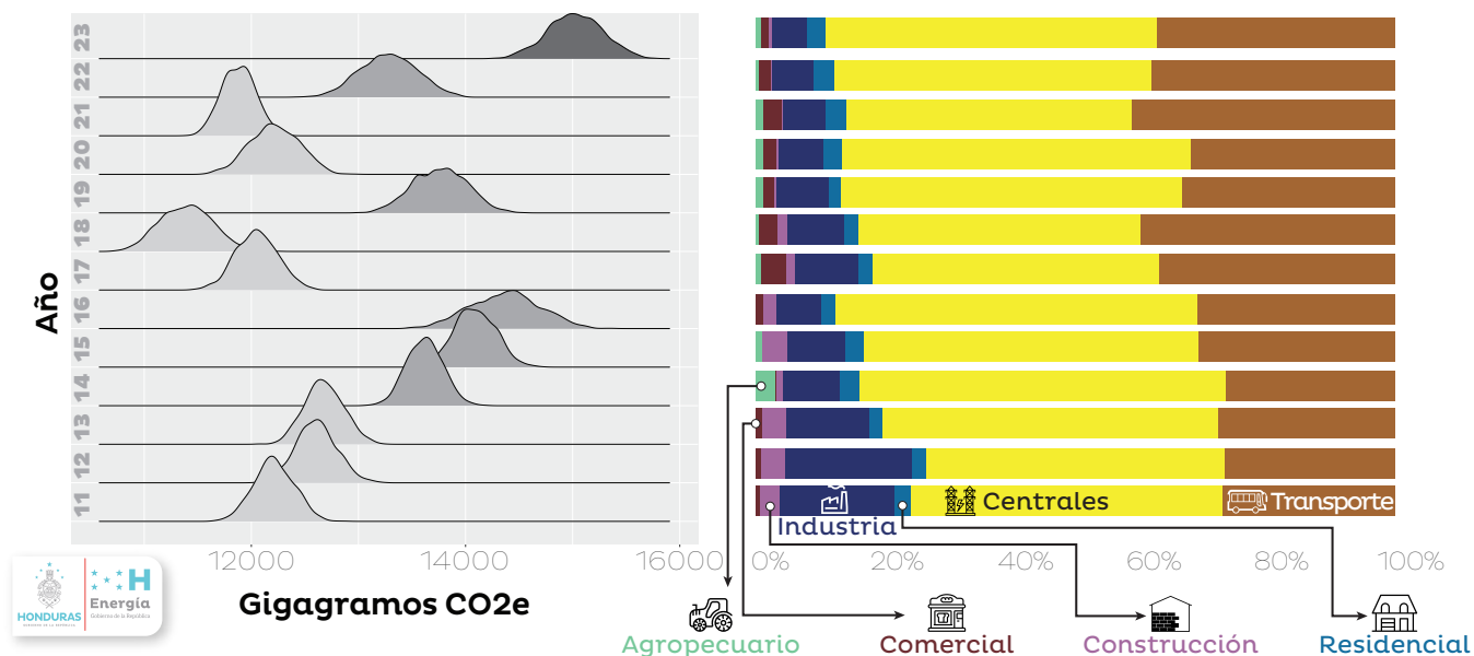
Figura 71. Emisiones de CO 2 e del sector energía 2011 - 2023
