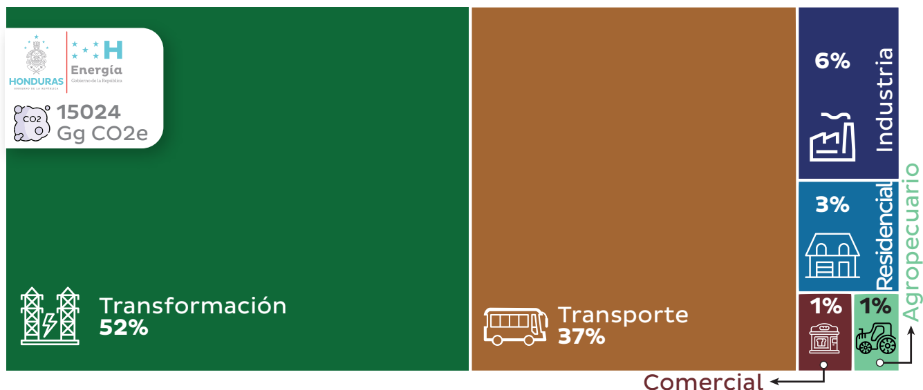
Figura 72. Emisiones de gases de efecto invernadero 2023, según sector de consumo
