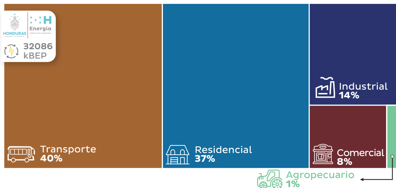
Figura 65. Demanda energética según sector de consumo durante el 2023
