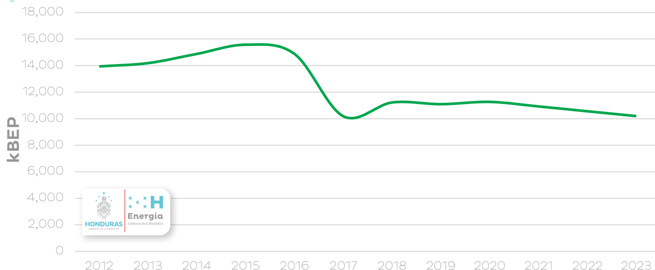
Figura 15. Producción de leña nacional durante 2012 – 2023
