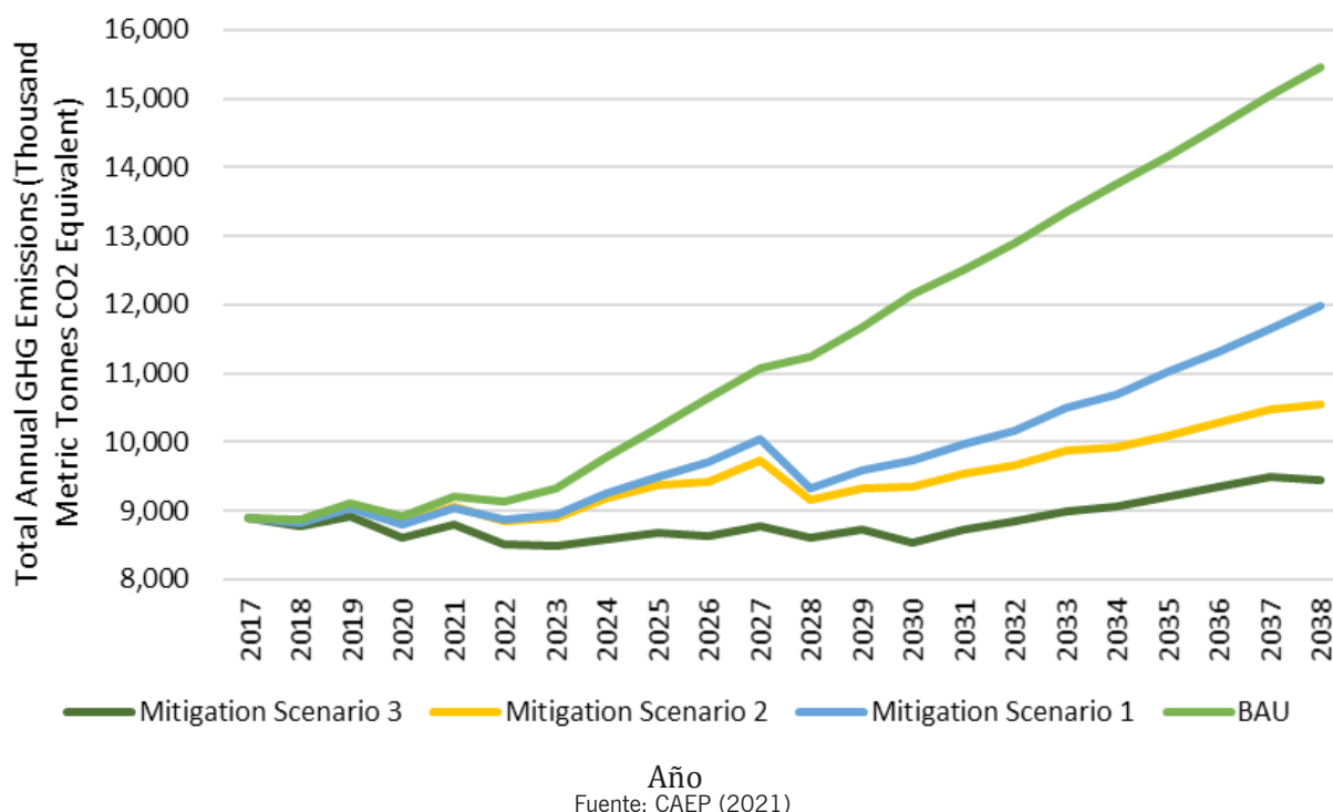
Figura 1 – Emisiones de GEI en los escenarios BaU y de mitigación para el sector de Energía
